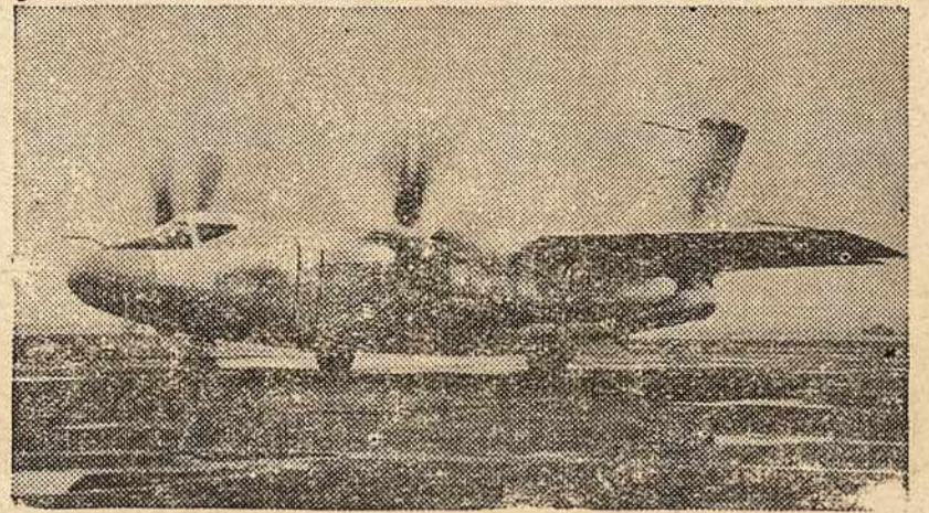
NAUJAS Amerikos bombardavimo lėktuvas XAAJ-1, sverias 26 toneladas ir yra sunkiausias lėktuvas, iš turinčių ant laivų lėštavnešių portoavionių. Per valandą greitį gali išvystyti ligi 650 klm.
