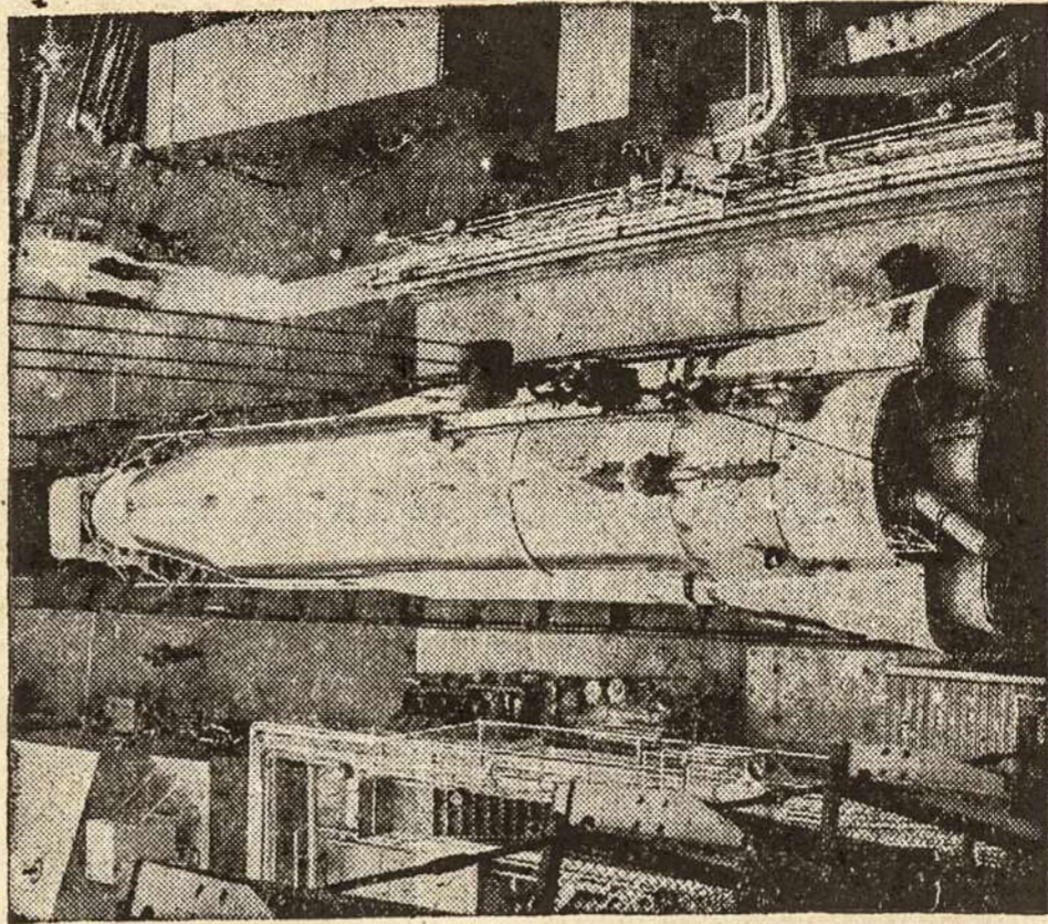
Balistinė «Atlas» bomba-raketa, 24 metrų ilgio ir 10 tonų svorio buvo išauta amerikonių Atlante. Jos greitumas per valandą siekia 24 tūkstančius 135 kilometrų. Ji nuskrido 4000 kilometrų. Ji stumiamą dviejų motorų, o trečias ją prilaiko.
