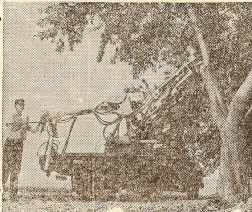
Amerikietis inžinierius agronomas demonstruoja praktiška medžių purtinimo mašiną, kuri yra įtaisyta suakvežimyje. Ji vartojama ypatingai rinkti almedroms.
