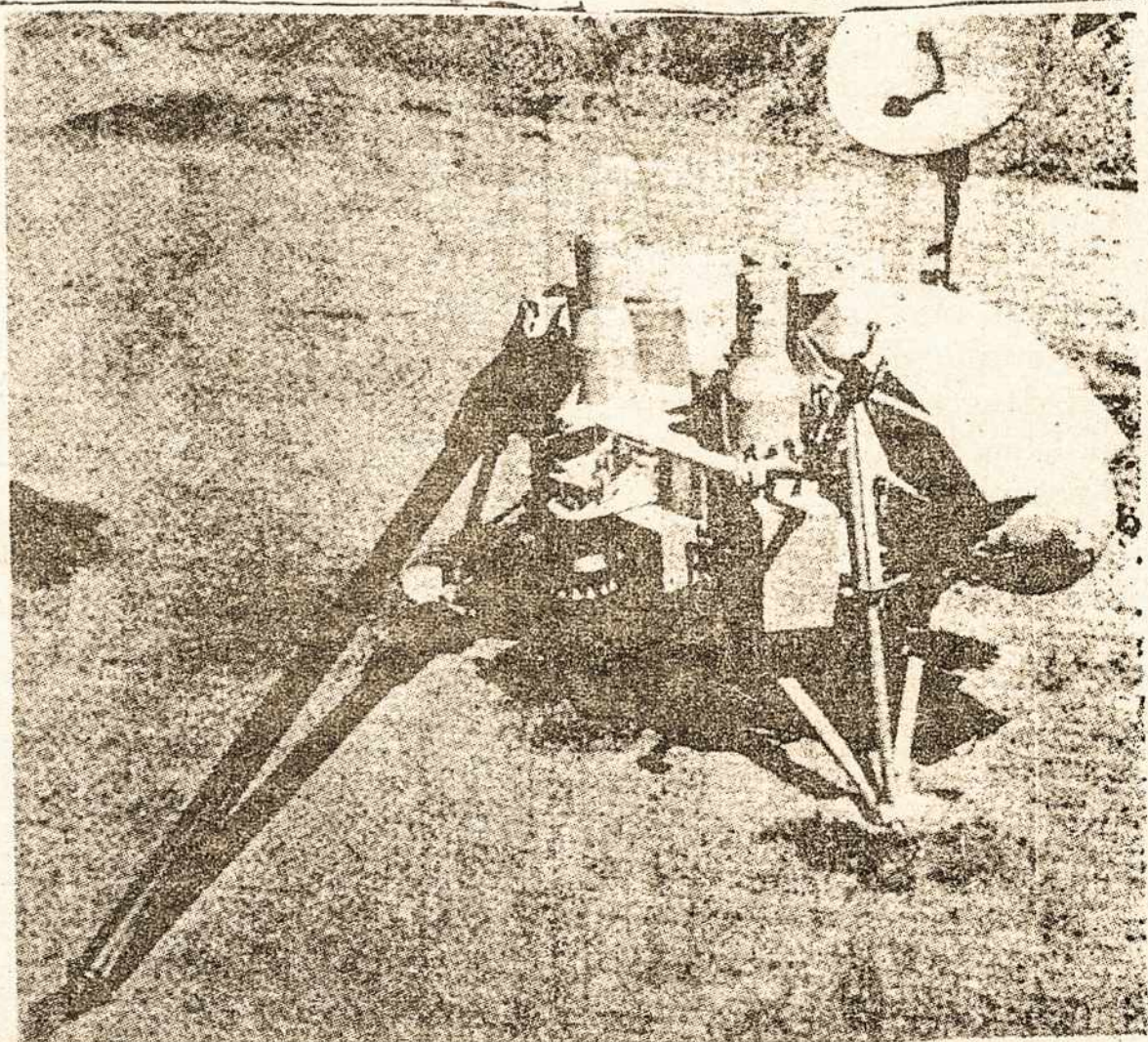
Toks aparatas yra nuleistas į Marso planetą. Tai mokslinė laboratorija, kuri tirs Marso planetos sudėtį. Kairėje matome ranką, kuri kasa žemę, paskui įtraukia į vidų ir išanalizuoja. Dešinėje aukštai — radijo antena.
