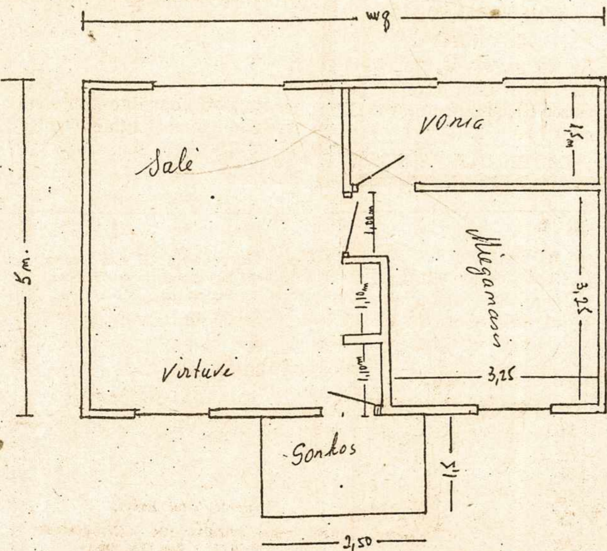
Pirmojo senelio namuko planas
