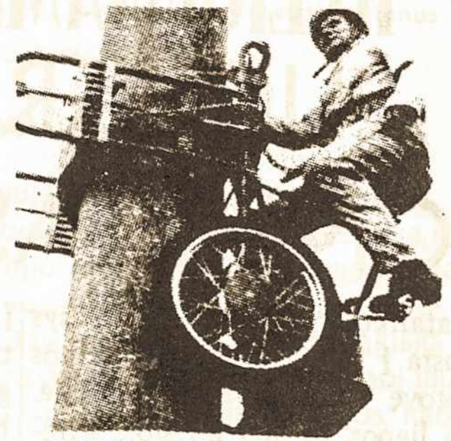
A BICICLETA-TREPADORA — O sr. V. tautas Gulbinas, professor de Mecânica na Politécnica de Kaunas, Lituânia, inventou a "bicicleta-trepadora", que pode subir nos postes. Na foto, o inventor com sua criação que pode subir até quinze metros, pedalando-se sem esforço, graças a um "artelho" de molas que "abraça" o poste.
