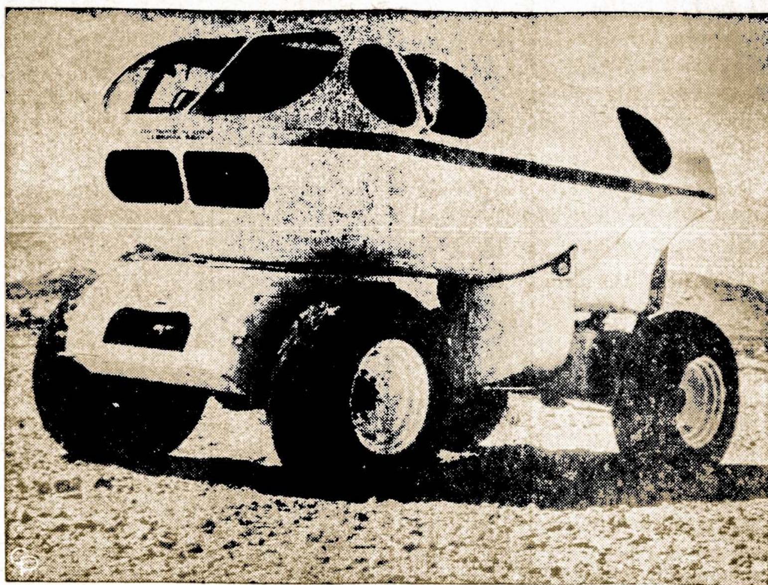
Geologinė laboratorija suprojektavo šį 8 tonų automobilį, kuriame įrengti instrumentai, kurie bus naudojami astronautams išsikėlus mėnulyje. Pietų Kalifornijos uolienų laukuose tie instrumentai išbandomi.
