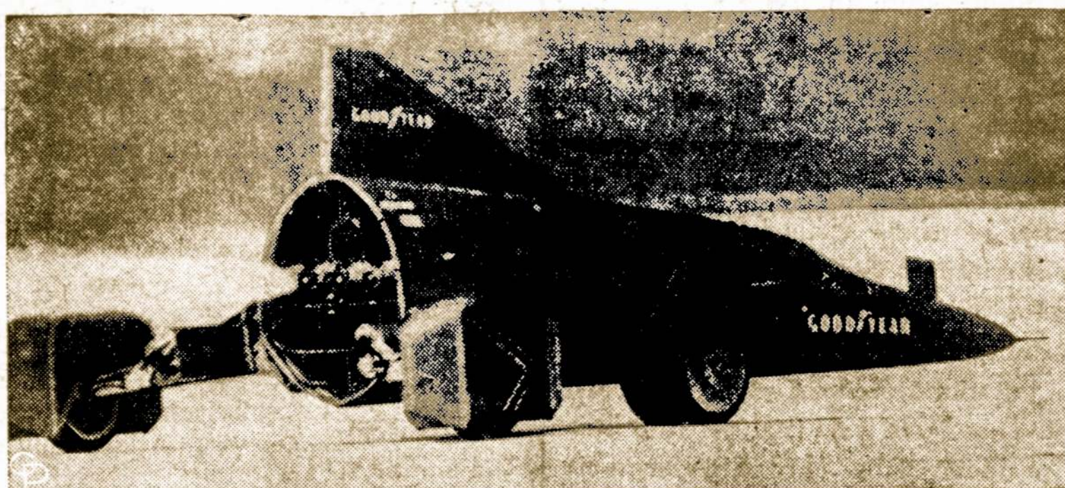
Tokio tipo automobilis, turis sprausminius motorus, išvystė žemėje didžiausią greitį, per valandą pasiekdamas, Bonneville, Utah, 536.71 mylių. Mašina turi 15 raketinių variklių ir rekordo siekiant buvo įjungta jų tik keturi. Vairavo Bob Tatroe.
