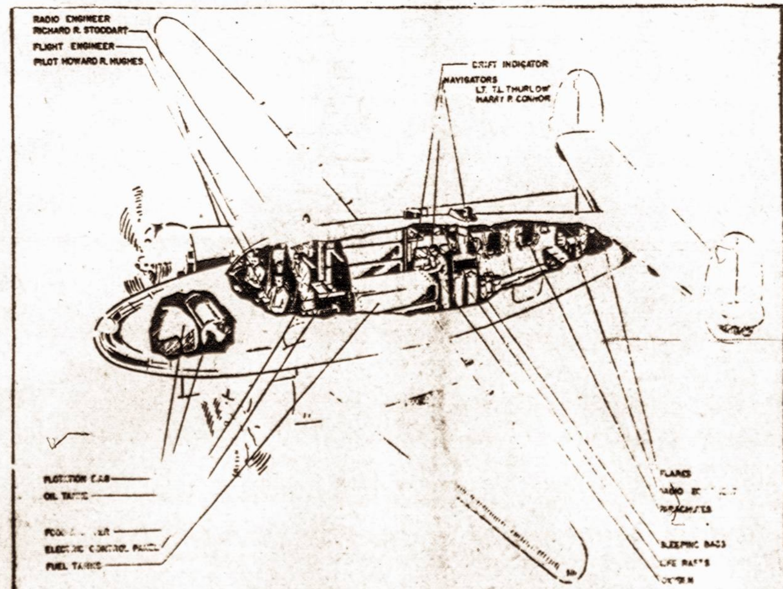
Patvarus lėktuvas skridimui aplink pasaulį. — Hovardo Hughes'o lėktuvas kainuoja 200,000 dolerių. Šiame plane parodytas lėktuvo suskirstymas. Kadangi jame yra daug naujų prietaisų, lėktuvas vadinamas skraidžiančiąja laboratorija.
