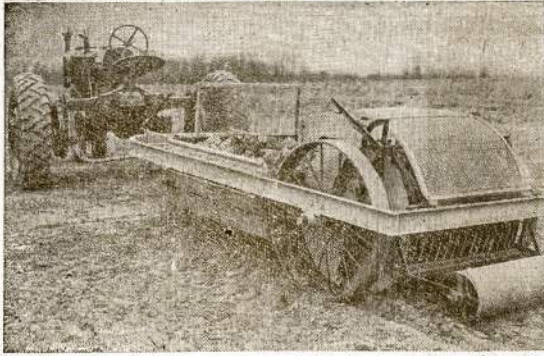
Dar tokios mašinos fermeriai neturėjo iki šiol. Tai akmenimis iš dirvų rinkti mašina. Ją neseniai išbandė Maine valstijoje, kur dirvoje randasi tiek jau daug akmenų, kaip ir Lietuvos laukuose. Mašina į vieną valandą gali surinkti 12-ą tonų akmenų.
