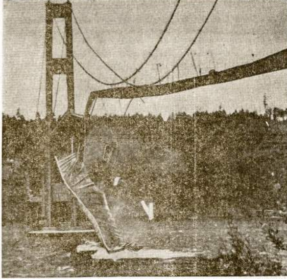
Nei šešis mėnesius neįstarnvęs sužlogo trečias pasaulį savo didumu plieninis tiltas netoli Seattle, Wash. Tiltas pataigtas statybių pereią liepos mėnesį ir sugruvijo šio mėnesio 7 dieną. Lėšavo $6,400,000. Daļ tēsu skyrē federālā valdžia. Vidurj dar ore bekabāncios tilto daļies matosi automobīlijus. Jo vairuotojas spējo išbēgti ir krantā.
