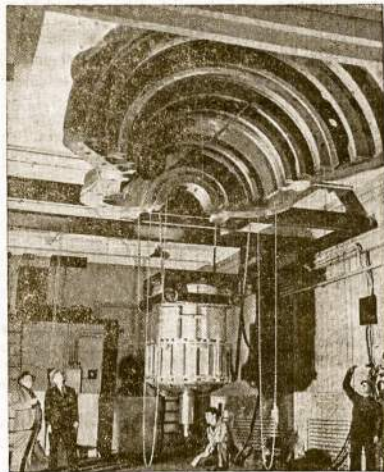
Naujausio modelio X-Ray foto aparatas, kurį šiom dienomis įsitaė General Electric korporacija savo laboratorijoj Schenectady, N. Y. Aparatas naudojamas fotografavimui plėninių masinių dalių. Jis peršviečia ir nufotografuoja 4 colių storio plėnė. Jei plėno šmote būtų koks netikslumas, kurio kitom priemonėm iš šiol nebūvo galima surasti, tai šis aparatas aiškiai tai parodo ant fotografijos.
