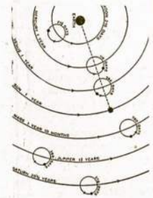
Ptolemajinė Sistema
