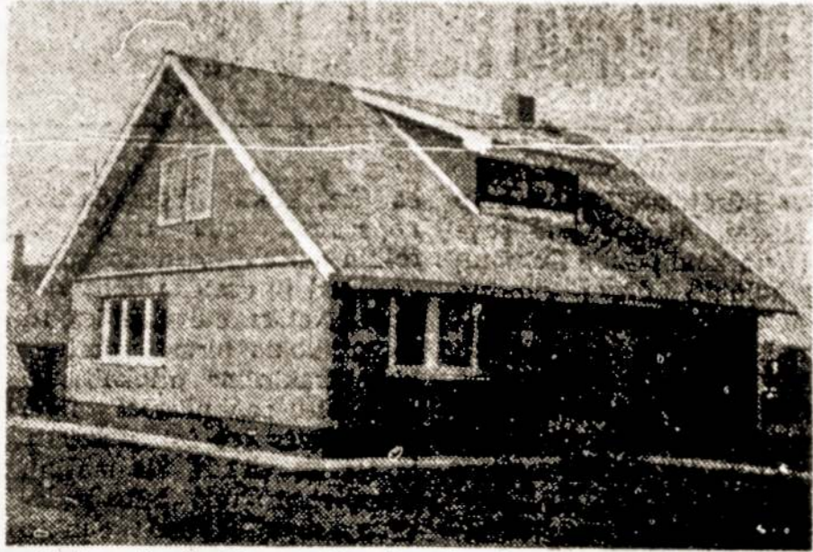
Eksperimentinis vienbutis, trijų kambarių namas iš keramzitoninio monolito, pastatytas Kabiškių gyvenvietėje.
