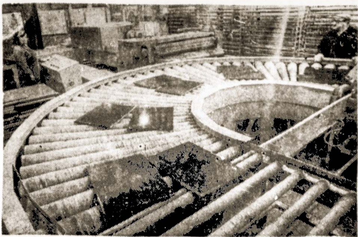
“Vilniaus” baldų kombinate pradėjo veikti pusiau automatine korpusinių detalių apdailos linija, kurią sukonstravo įmonės specialistai. Jos pajėgumas — 6-8 tūkstančiai detalių per pamainą.
