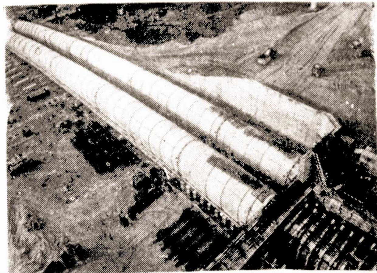
Kaišiadorių hidroakumuliacinės elektrinės statyboje montuojamas didelio skermens vamzdynas [nuotraukoje], kuriuo bus keliamas vanduo iš Kauno marių. V. Usinavičiaus nuotr.
