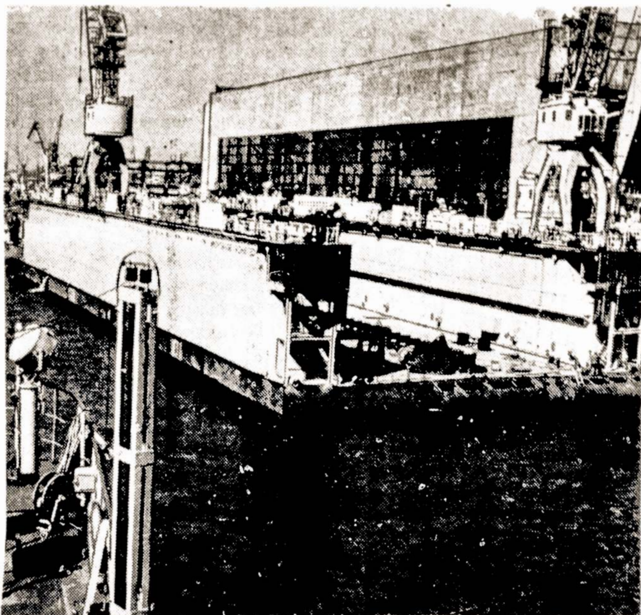
Klaipėdos "Baltijos" laivų statyklos pastatyti plaukiojantys dokai gerai vertinami įvairiose pasaulio šalyse. Neseniai čia baigtas statyti autonominis 4,500 tonų keliamosios galios plaukiojantis dokas Kubai. Tai ketvirtas toks dokas šios šalies remontininkams. Šiuo metu dokas jau perduodamas užsakovams. B. Aleknavičiaus nuotr.
